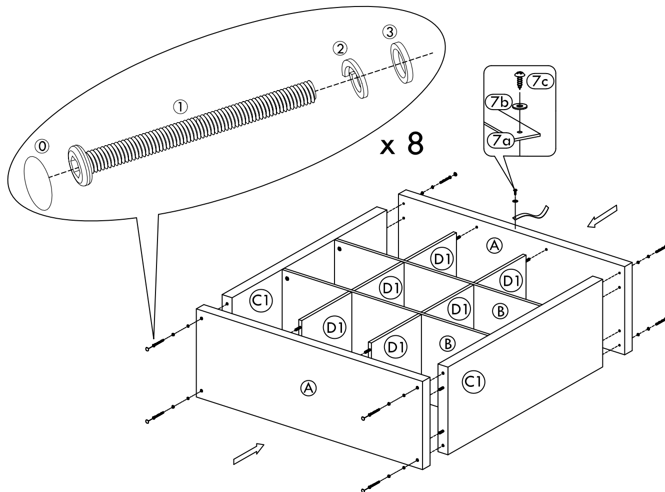
Tornillo
