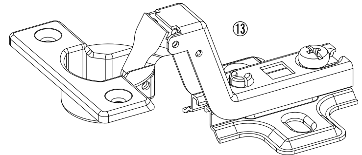
Hinges Qty: 4
