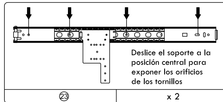
Diapositiva del cajón 2
