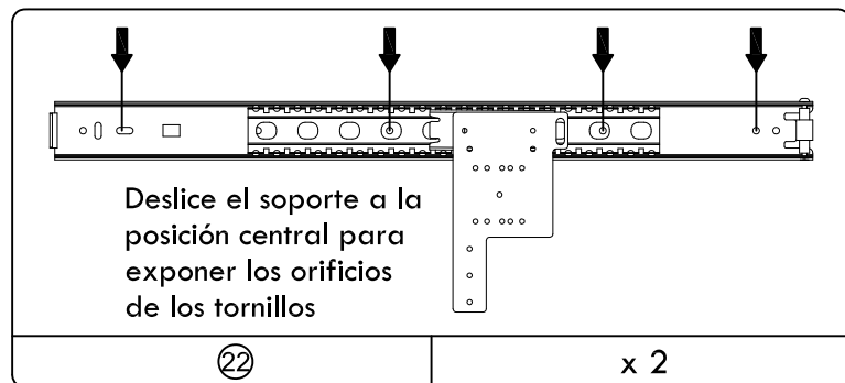
Diapositiva del cajón 1
