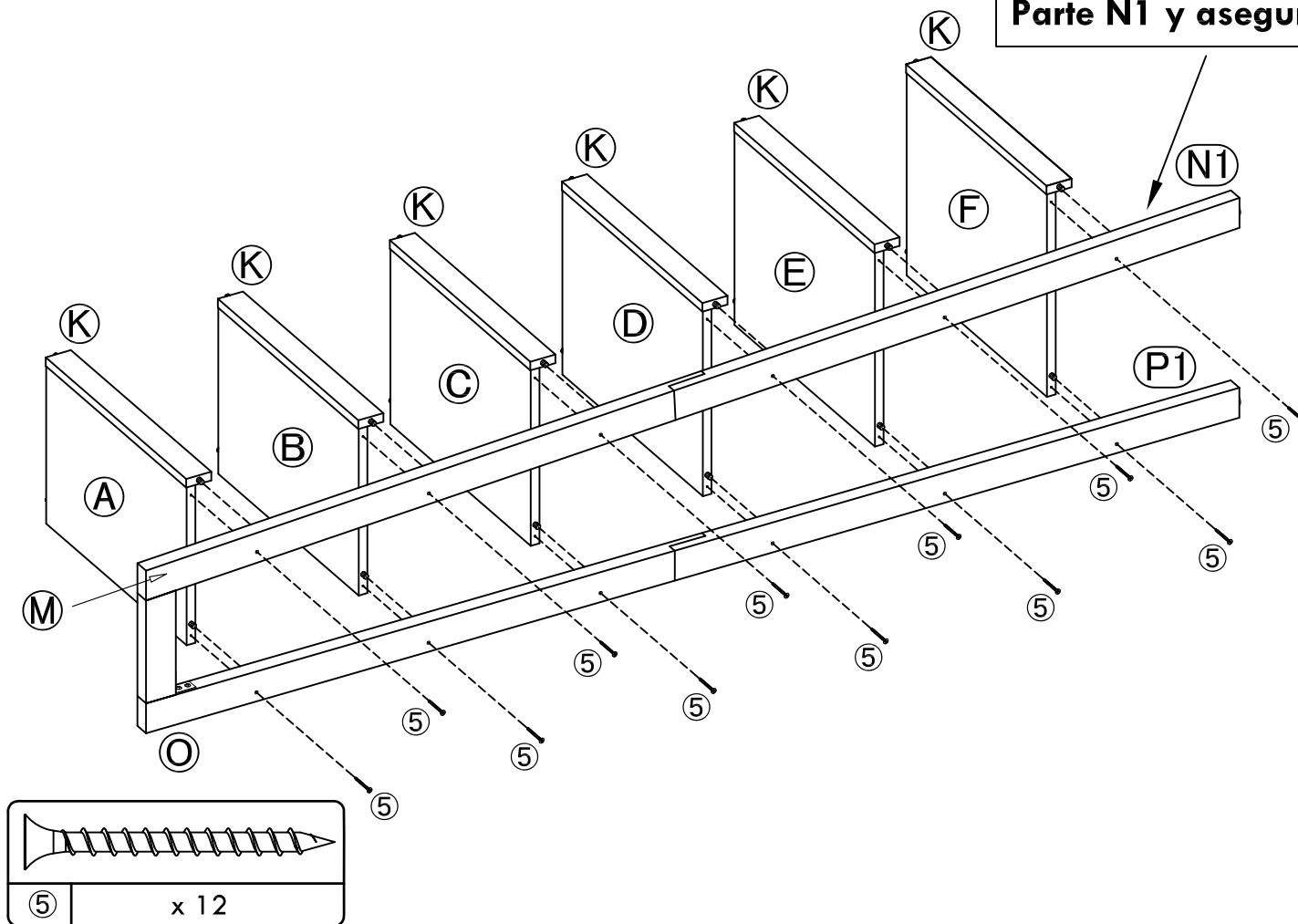
Tornillo 1
