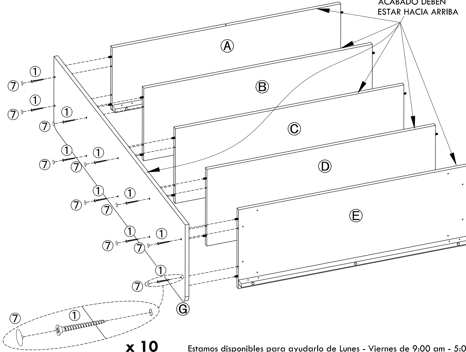
Tornillo 1
