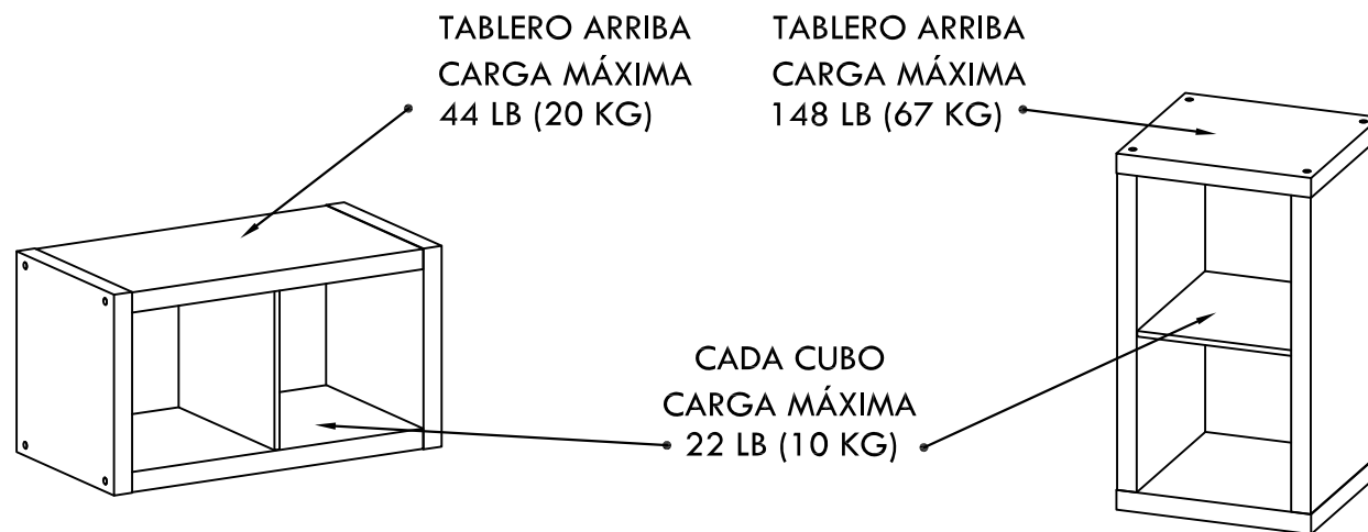
CONFIGURACIÓN OPCIONAL
