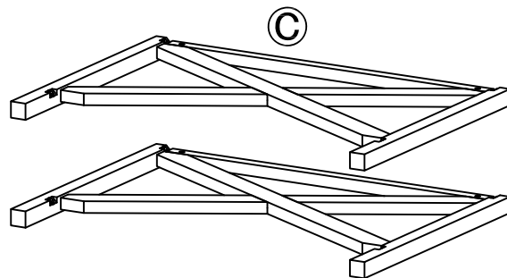
Marco de lateral (Cantidad: 2)
